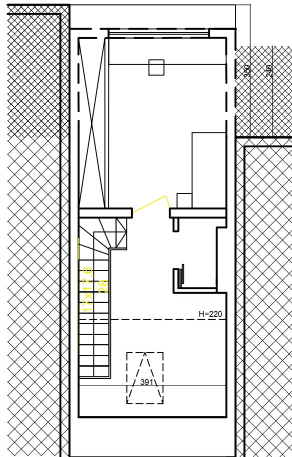
PODDASZE
